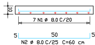
Base em concreto armado
