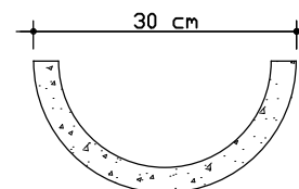
Canaleta de escoamento de água
