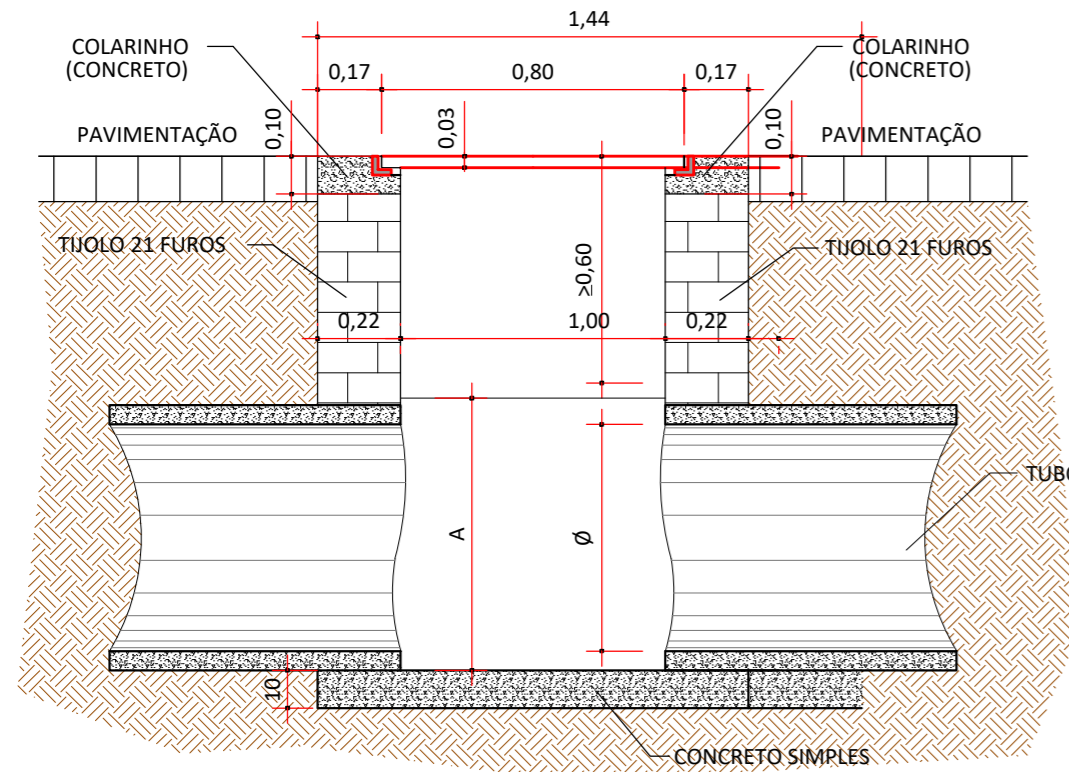
CORTE LONGITUDINAL (A A)
