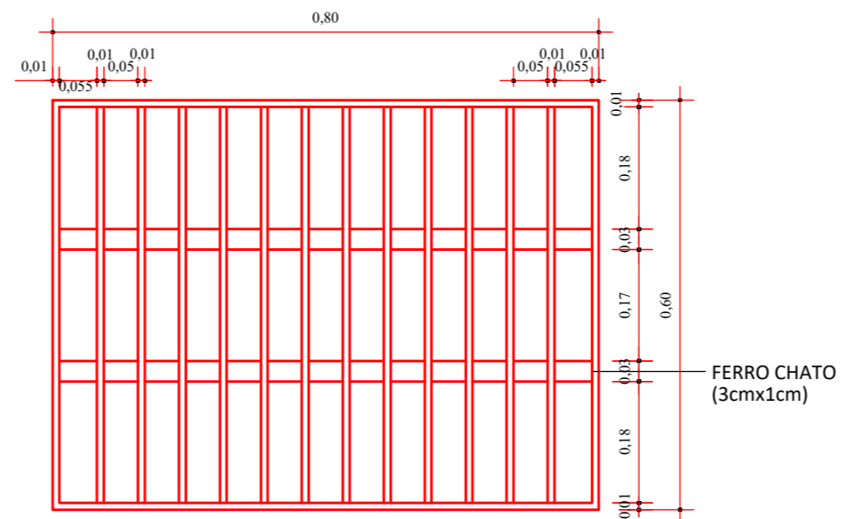
PLANTA - GRELHA
